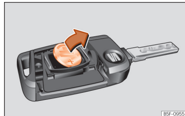
Slika 46 Ključ vozila: odstranjevanje baterije.
