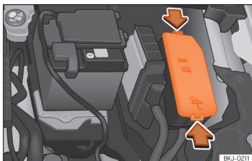
Slika 168 V motornem prostoru: pokrov postaje z varovalkami.
