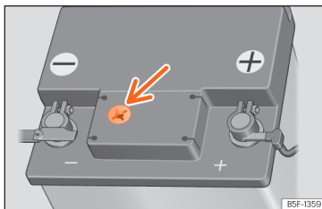
Slika 187 Vidno okence na zgornji strani 12-voltnega akumulatorja (shematski prikaz).
