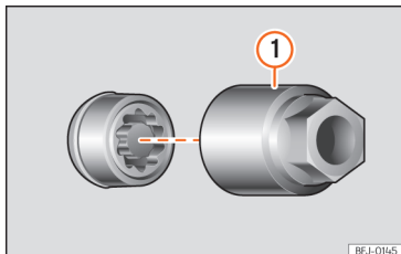
Slika 194 Kolesni vijak z zaščito pred krajo, zaščitni pokrovček in adapter.
