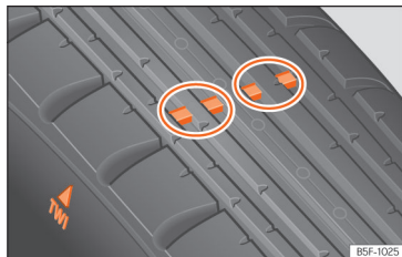
Slika 189 Profil pnevmatike: oznake obrabljenosti
