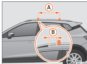
Slika 147 Pritrdilne točke prečnih nosilcev za strešni prtljažnik.
