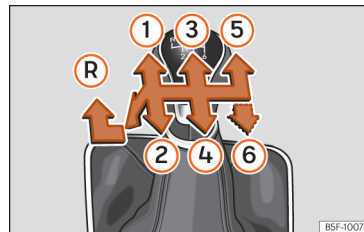
Slika 84 Prestavna shema pri 5- oz. 6-stopenjskem ročnem menjalniku
