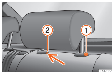
Sl. 110 Zadnji vzglavnik: demontaža
