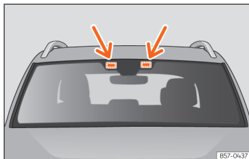
Sl. 137 Območja za namestitev elektronskih dodatkov.
