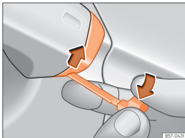
Sl. 83 Kljuka voznikovih vrat: odstranitev pokrova
