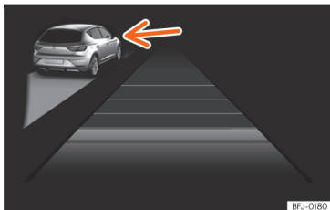
Sl. 170 Na zaslonu kombiniranega instrumenta: ACC aktiven, zaznano vozilo na levi strani
