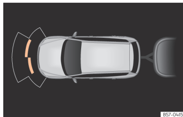
Sl. 193 Prikaz parkirne asistencije na zaslonu s priklopljeno prikolico
