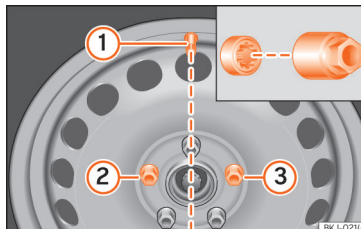
SL. 37 Menjava kolesa: ventil pnevmatike ① in ustrezni mesti za namestitev vijaka z zaščito pred krajom ② ali ③.
