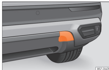
Sl. 47 Zadnji odbijač, desna stran: odstranjanje pokrovčka.
