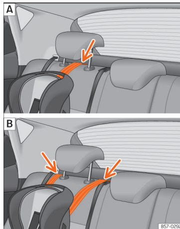
Sl. 28 Zadnji sedež: nastavev in vgradnja glede na pas Top Tether.
