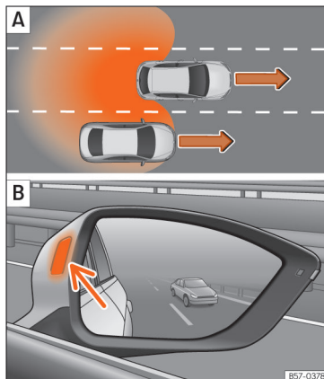
Sl. 180 Shematski prikaz: [A] Postopek prehitevanja in nato menjava na desni vozni pas. [B] Prikaz asistencije za opozarjanje na vozila v mrtvem kotu v desnem zunanjem ogledalu.
