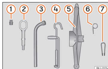
Sl. 31 V prtljažniku pod dnem prtljažnika: avtomobilsko orodje.
