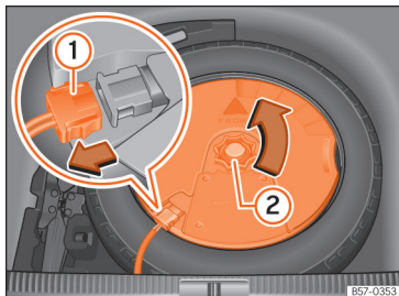
Sl. 223 V prtljajniku: demontaža globokotonskega zvočnika.
