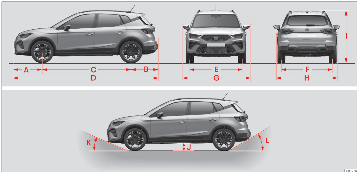
Slika 205 Mere in koti
