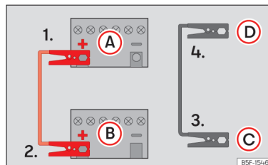
Slika 161 Načrt priključitve za vozila s sistemom start-stop.
