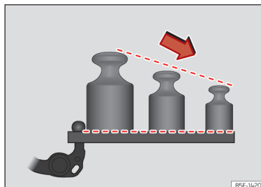
Slika 149 Priporočena porazdelitev mase na sistemu nosilcev zadaj.
