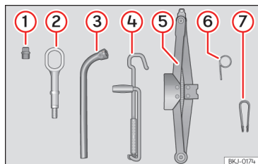
Slika 156 V prtljajniku pod dnom prtljažnika: avtomobilsko orodje.
