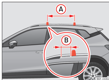
Slika 147 Pritrdilne točke prečnih nosilcev za strešni prtljajnik.
