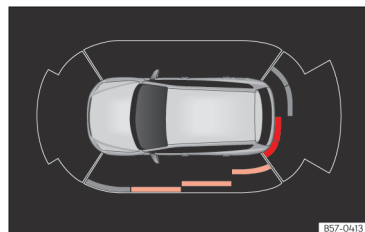
Slika 121 Prikazi parkirne krmilne asistencije na zaslonu infotainment sistema.
