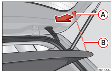
Slika 142 V prtljažniku: odstranjevanje in nameščanje zadnje police
