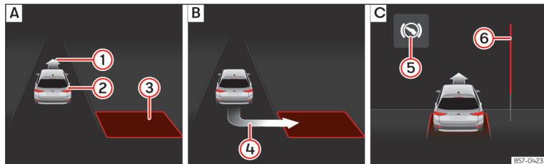
Slika 127 Na zaslonu kombiniranega instrumenta: prečno parkiranje. [A]: Iskanje prostega parkirnega mesta [B]: Parkirni položaj. [C]: Maneviranje.
