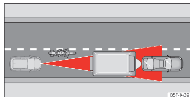
Slika 105 Spredaj vozeči motorist prehitava zunaj območja dosega radarskega senzorja.
