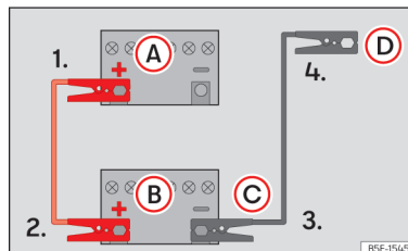
Slika 160 Načrt priključitve za vozila brez sistema start-stop.
