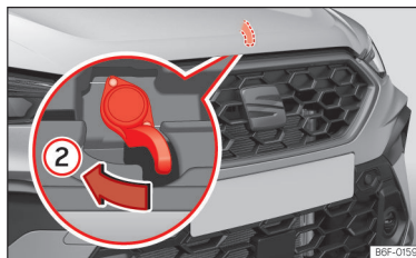
Slika 178 Ročica pod pokrovom motornega prostora.
