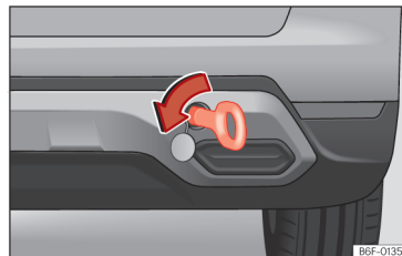
Slika 166 Na desni strani zadnjega odbijača: privito vlečno uho.
