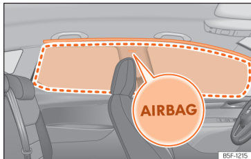
Slika 31 Mesto vgradnje in območje delovanja varnostne blazine za glavo.
