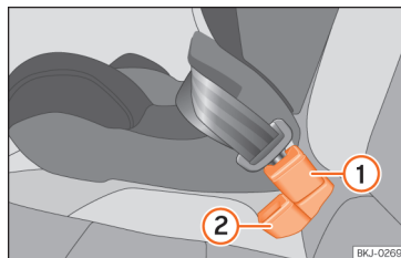
Slika 40 Položaj zaklepov varnostnih pasov na zadnji sedežni klopi
