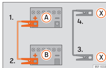
Slika 162 Načrt priključitve za vozila s sistemom start-stop.
