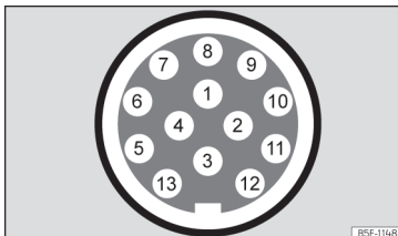
Slika 149 Shematski prikaz: dodelitev konektorskih zatičev za električni tok prikolic
