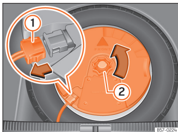
Slika 192 V prtljažniku: odstranite globokotonski zvočnik
