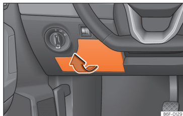
Slika 168 Na voznikovi strani armaturne plošče: pokrov postaje z varovalkami.
