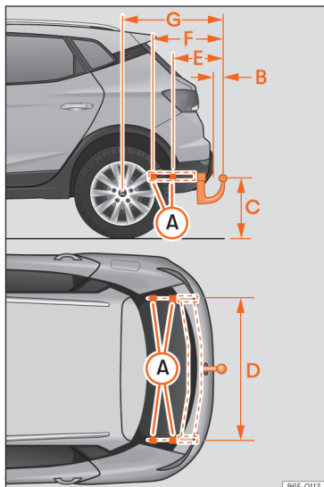
Slika 152 Mere in pritrdilne točke za naknadno vgradnjo vlečne naprave
