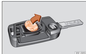
Slika 46 Ključ vozila: odstranjevanje baterije.
