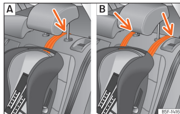
Slika 38 Zadnji sedež: nastavitev in vgradnja glede na pas Top Tether.
