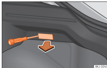
Slika 176 Osvetlitev prtljažnika.
