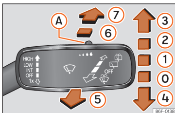
Slika 72 Upravljanje naprave za brisanje vetrobranskega in zadnjega stekla.
