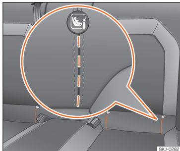
Slika 35 Zadnji sedež: izrezi za dostop do sidrnih točk sistema ISOFIX/i-Size.
