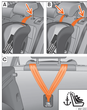
Sl. 34 Zadnji sedež: nastavitev in vgradnja glede na pas Top Tether.
