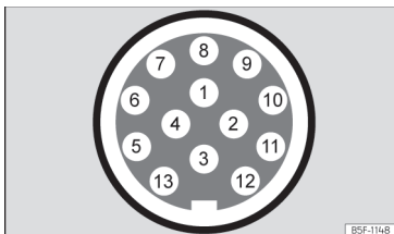
Sl. 206 Shematski prikaz: dodelitev konektorskih zatičev v električni vtičnici za prikolico.
