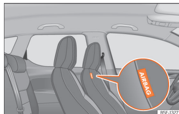
Sl. 24 V blazini sedežnega naslonjala voznikovega sedeža: sredinska varnostna blazina.
