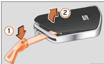
Sl. 84 Ključ vozila: odpiranje pokrova predalčka za baterijo.
