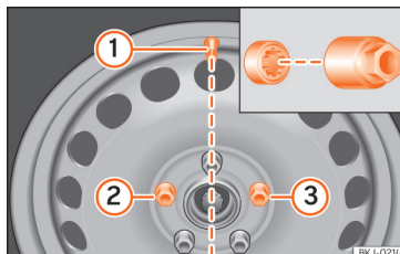
Sl. 44 Menjava kolesa: ventil pnevmatike ① in ustrezni mesti za namestitve vijaka z zaščito pred krajom ② ali ③.
