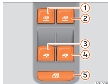
Sl. 99 Del vozniških vrat: elementi za upravljanje električnega pomika sprednjih in zadnjih stekel
