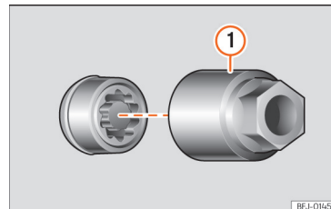
Sl. 42 Kolesni vijak z zaščito proti kraji, zaščitni pokrovček in adapter.
