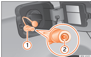
Sl. 222 Odprta loputa rezervoarja: odprtina za točenje plina (1), nastavak za točenje plina (2).
