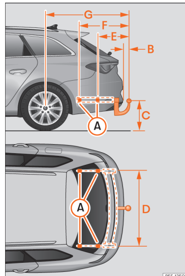
SI. 208 Mere in pritrdilne točke za naknadno vgradnjo vlečne naprave
